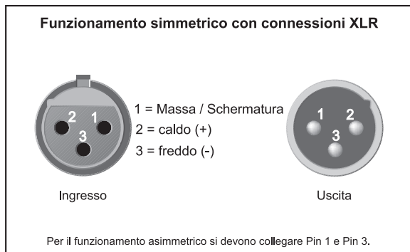
Fig. 7.3: Connettori XLR
