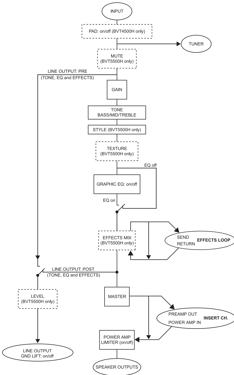
Fig. 8.1: schema a blocchi del BVT4500/5500H (I rettangoli rappresentano i comandi, gli ovali rappresentano i jack.)
