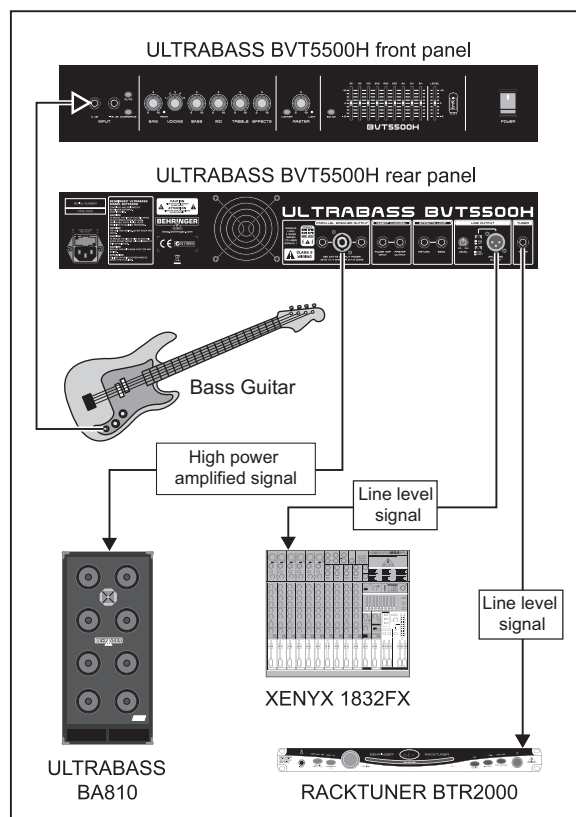
Fig. 5.1: esempio di configurazione del BVT5500H
