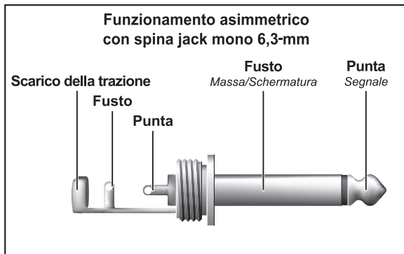
Fig. 7.1: Presa jack mono da 6,3 mm
