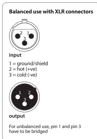
Fig. 4.1: Connettori XLR
